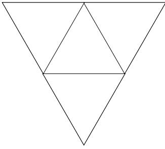
viervlak
