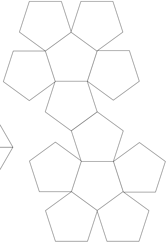
twaalfvlak
