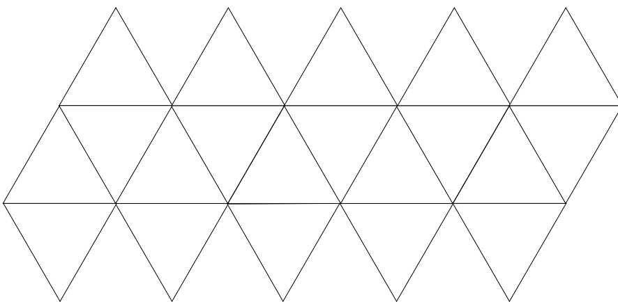
twintigvlak
